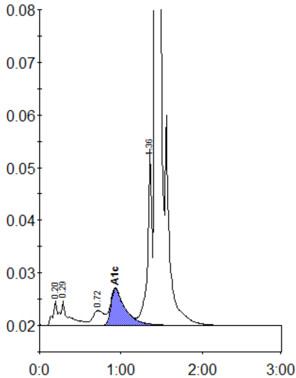
Peak table - ID: 10491229
